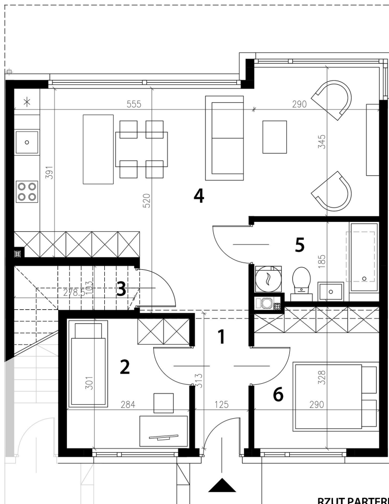
RZUT PARTERU
